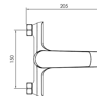
Ref. 121423 Monomando baño ducha Bathtub mixer Acabado cromo Cartucho 25 mm
