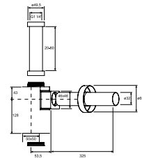
Ref. 123501 Sifón telescópico de lavabo Cuadrado 1"¼ latón. Cromo
