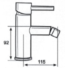
Ref. 121102 Monomando bidé Bidet Mixer Acabado cromo Cartucho 35 mm
